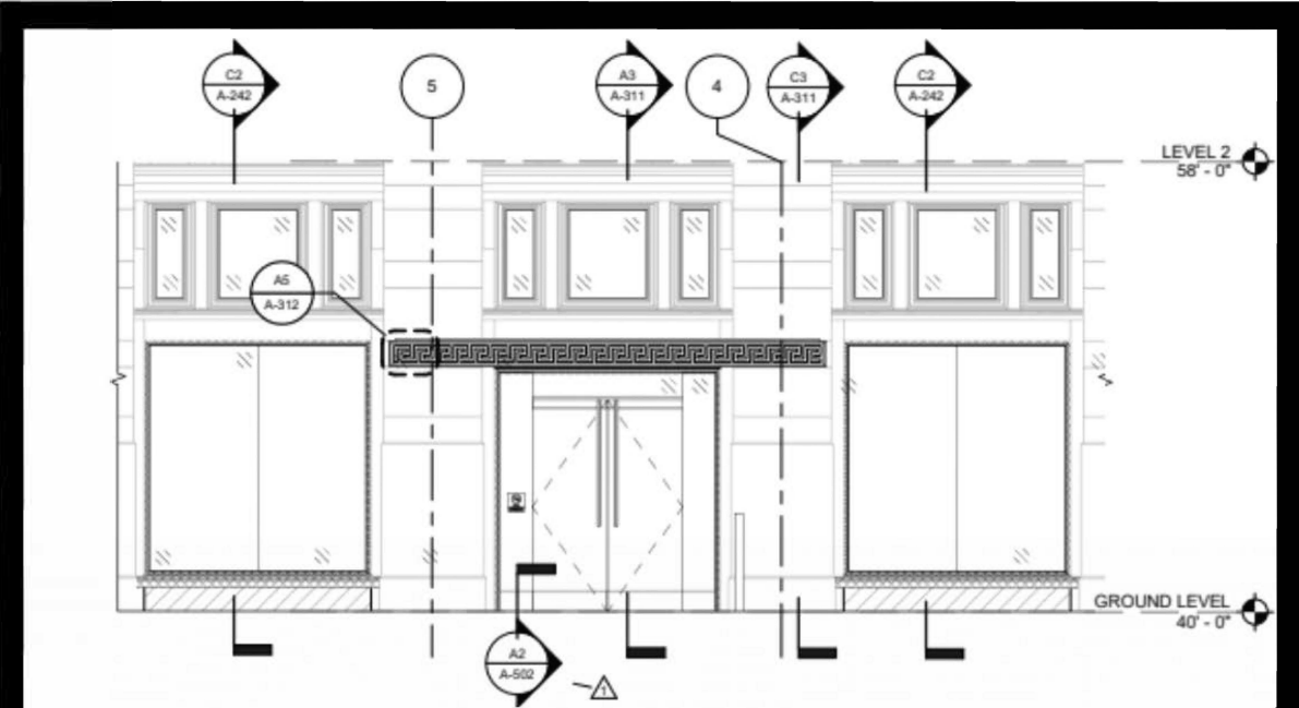
D1 ELEVATION - MARQUEE FRONT Scale: 1/4" = 1'-0" C1, A-212
