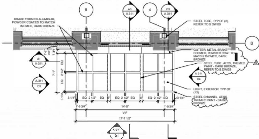
C1 RCP - MARQUEE Scale: 1/4" = 1'-0" A1, A-021
